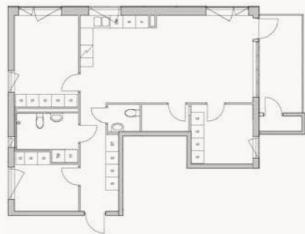
FYRRUMSLÄGENHET
